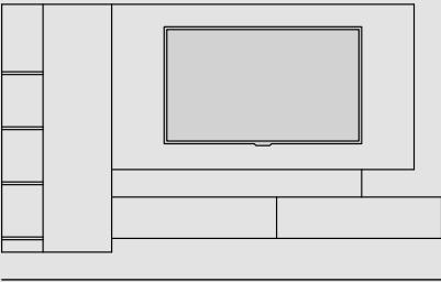
Skyline 25 layout 03 Variante C L.320 H.180 P.34/46 / W.320 H.180 D.34/46
